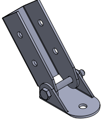
Ayarlanabilir Açılı Braket Adjustable Bracket Sayfa / Page 25
