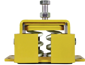
VibraPLUS-4 Yaylı Sismik İzolatör VibraPLUS-4 Seismic Vibration Isolator Sayfa / Page 108
