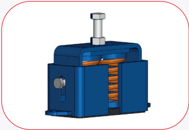
VibraTECH-2 Yaylı Sismik İzolatör VibraTECH-2 Seismic Vibration Isolator
