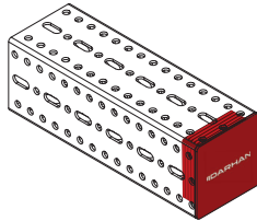
Profil Kapağı - DEC End Cap - DEC
