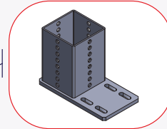
Köşe Bağlantı Adaptörü - DFL Angle Fitting - DFL
